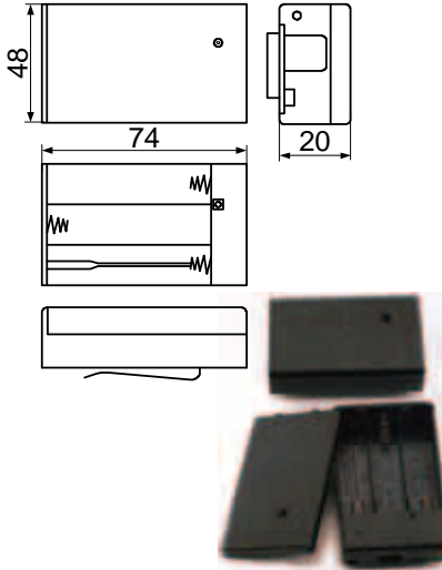
SBH-331-1A SBH-331-1AS
