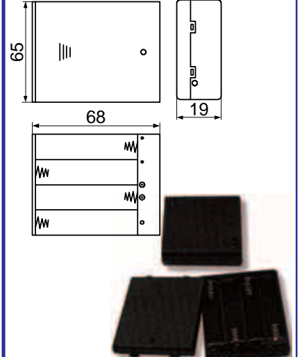
SBH-341-1A SBH-341-1AS
