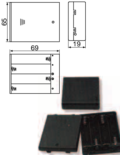
SBH-341A SBH-341AS
