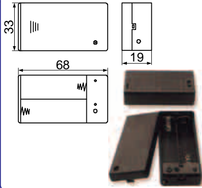
SBH-321-2A
