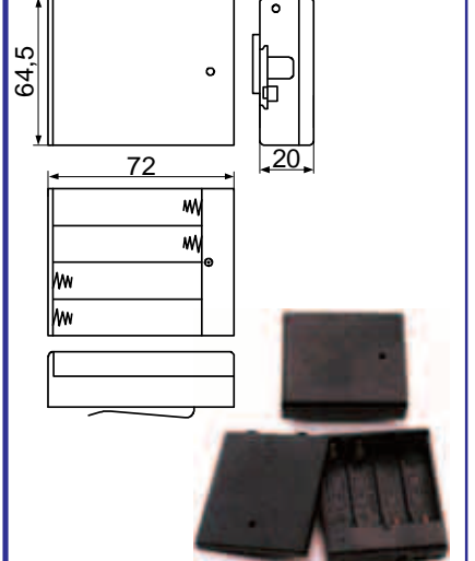
SBH-341-2A SBH-341-2AS
