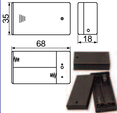
SBH-321-3A SBH-321-3AS
