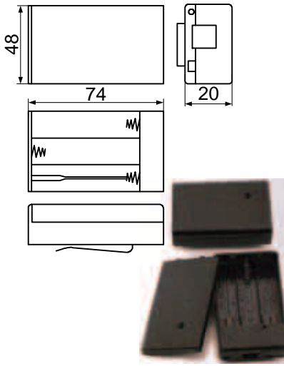
SBH-331-2A SBH-331-2AS
